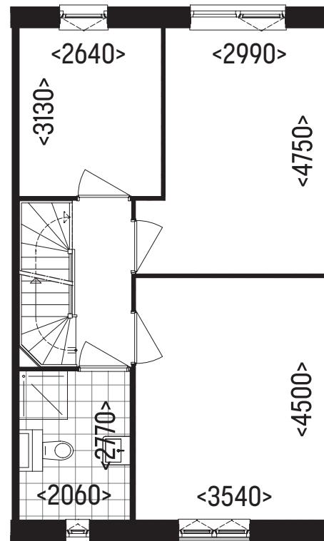
Eerste verdieping
